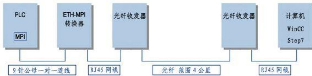
S7-300PLC与上位机远程连接示意图
